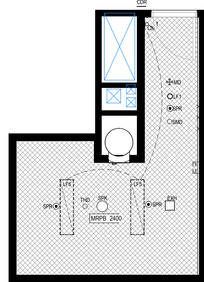
8 RCP-SLUICE Scale 1 : 50
